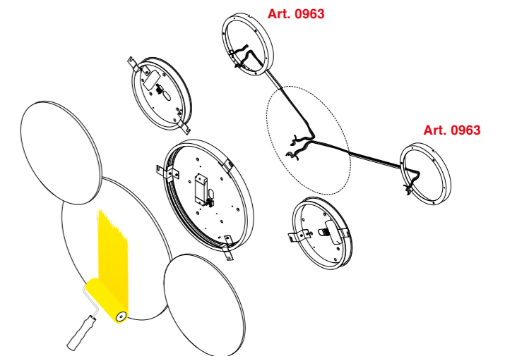
Esempio di installazione multipla con distanziali. Example of multiple installation with spacers.
